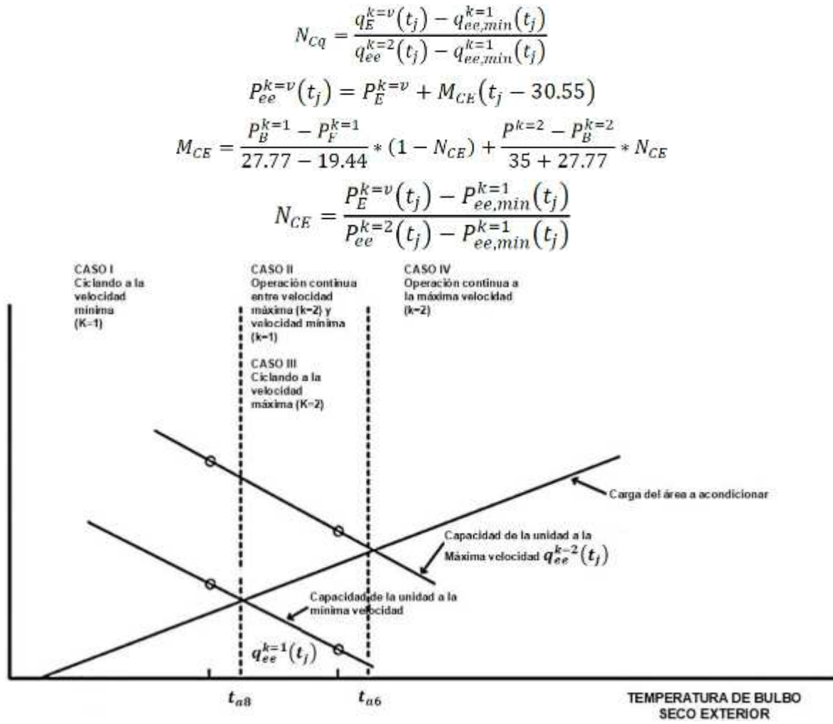
Figura 1a - Diagrama esquemático de varios modos de operación para la unidad INVERTER en modo frío
