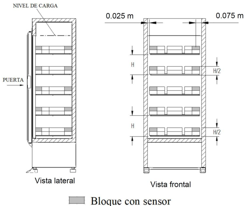
Figura E.15 - Colocación de bloques con sensor en congelador vertical
