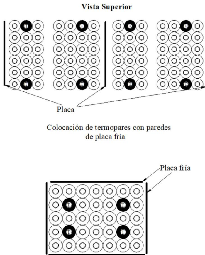
Figura E.14 - Colocación de sensores en enfriador horizontal de placa fría vista superior
