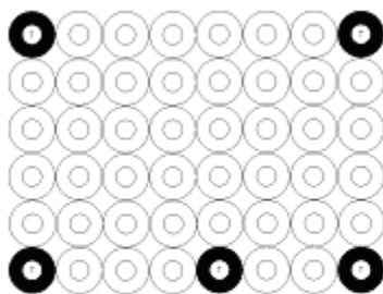
Figura E.5 - Colocación correcta de sensores de prueba en parrillas
