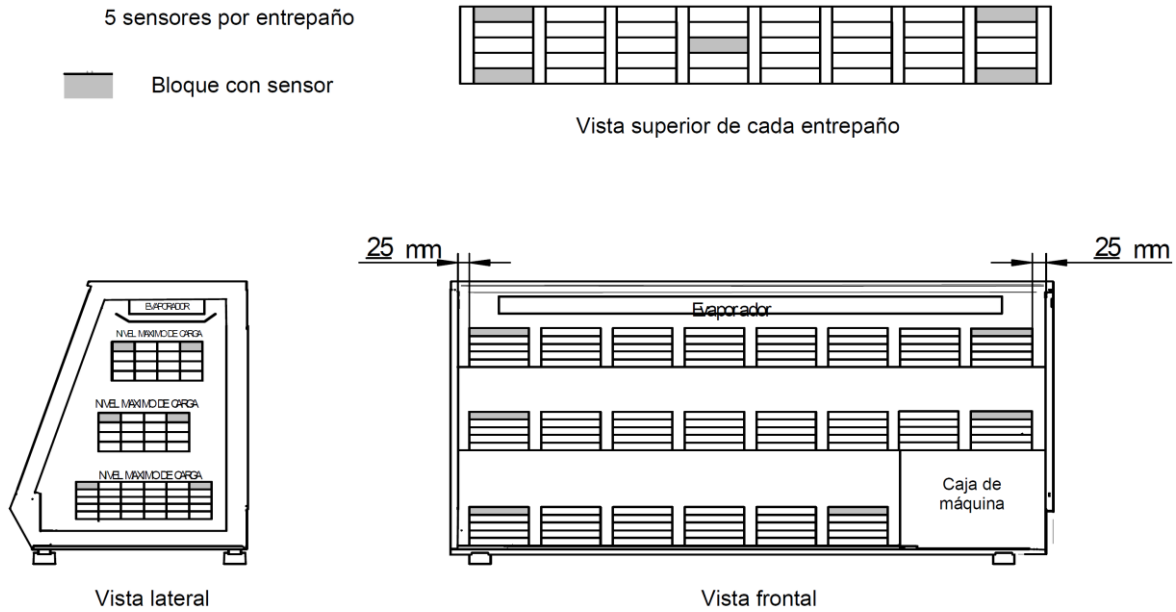
Figura E.17 - Colocación de bloque con sensor en vitrina refrigerada cerrada con puertas
